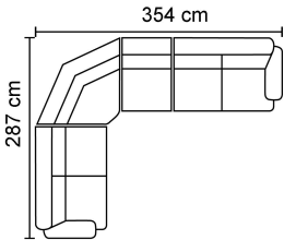
002 SECT.(16+29+01+17)
